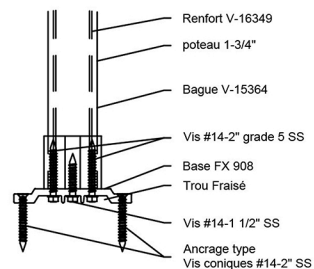
Base FX Vue en Élévation
