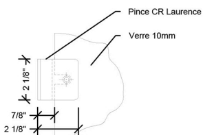
Pince CR Laurence Vue en Plan
