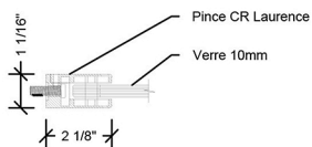
Pince CR Laurence Vue en Plan
